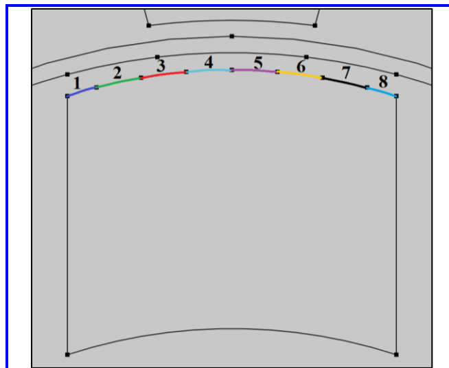
Рис. 3. Распределение потерь на вихревые токи в постоянном магните, а также в стали якоря и ротора
