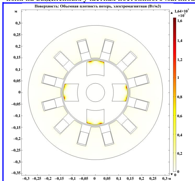
Рис. 5. Распределение потерь на вихревые токи в постоянных магнитах
