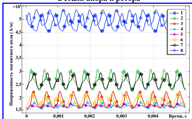
Рис. 4. Распределение напряженности магнитного поля на выделенных участках постоянного магнита
